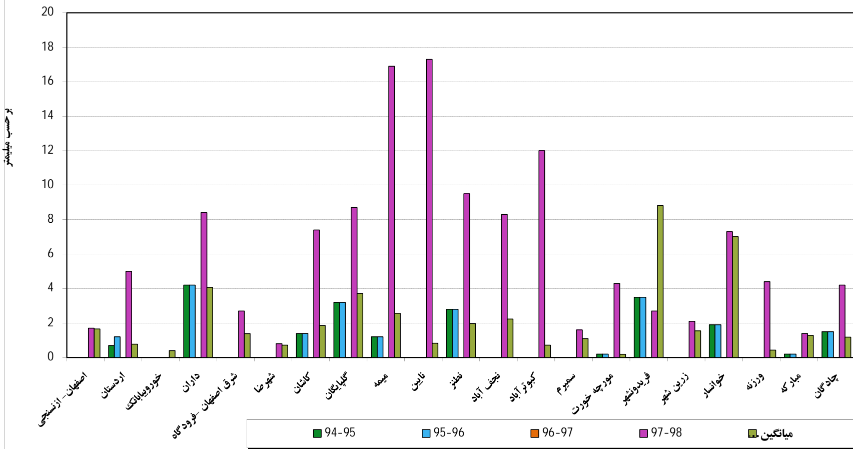
نمودار بارندگی سال زراعی جاری و مقایسه آن با سال های قبل تا ساعت 10:30 صبح مورخه 1397/07/28
