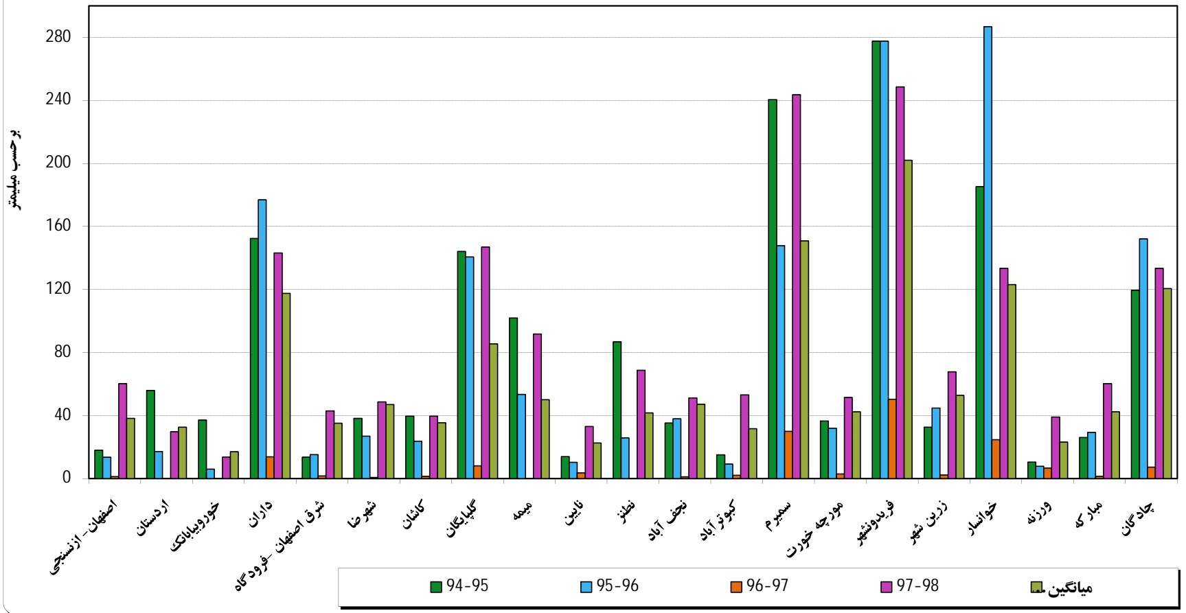
نمودار بارندگی سال زراعی جاری و مقایسه آن با سال های قبل تا ساعت 10:30 صبح مورخه 1397/10/15
