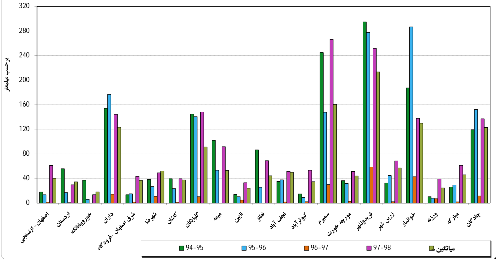
نمودار بارندگی سال زراعی جاری و مقایسه آن با سال های قبل تا ساعت 10:30 صبح مورخه 1397/10/18
