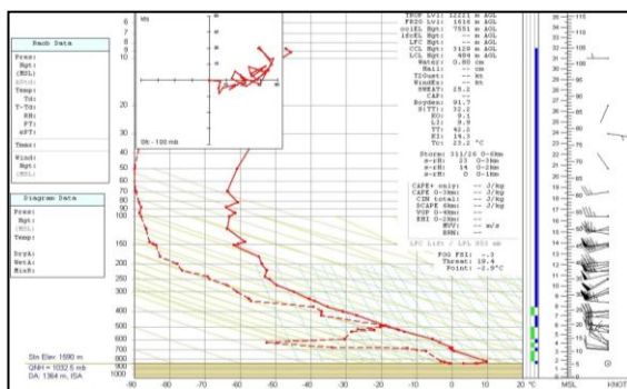
شکل ۷- نمودار skew-t-اصفهان روز ۱۹ آبان ۱۳۹۵ در ساعت ۰۰:۰۰ گرینویچ
